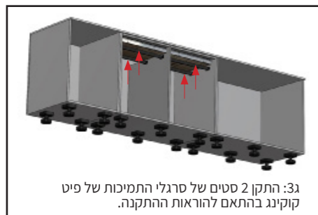
3ב: התקן 2 סטים של סרגלי התמיכות של פייט קוקינג בהתאם להוראות ההתקנה.
